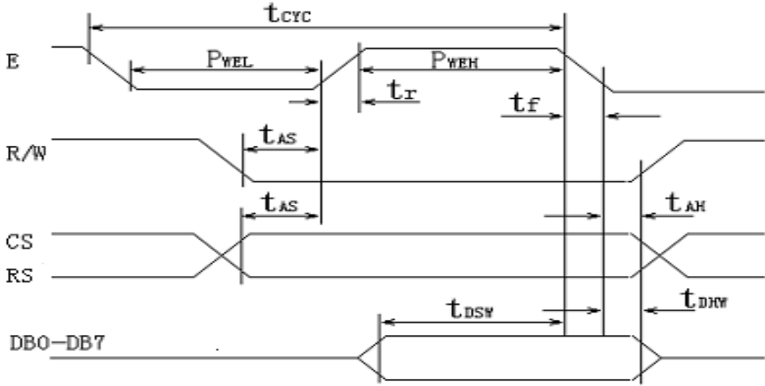
时序 1
