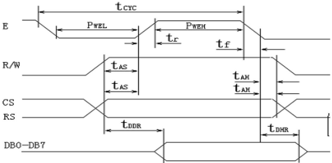
时序 2
